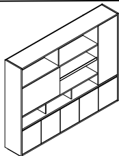
名称: 品毅A款文件柜 型号: PNY-CAA-2419 规格: 2400W*400D*1900H
