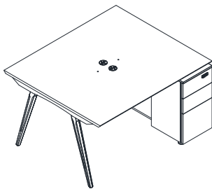
名称: 品毅B款两人位 型号: PNY-WTB2-1212/1412 规格: 1200W*1200D*750H 1400W*1200D*750H
